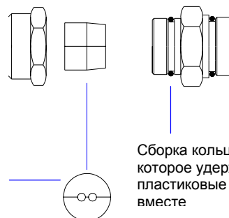
Адаптер KDO832 для введения двух 3 мм волокон
