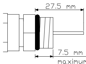
Рис. 3. Разъем ВЧ кабеля
